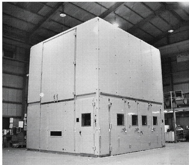
プレス機の騒音を防ぐ防音BOX
